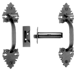
WTXBI Mortise Latch
